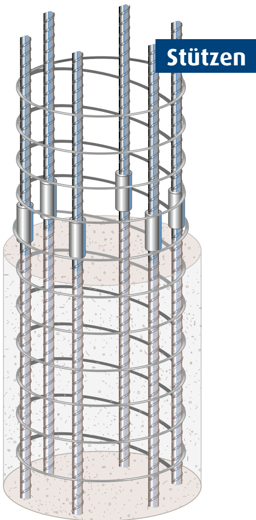
Mit Schraubmuffenverbindungen
